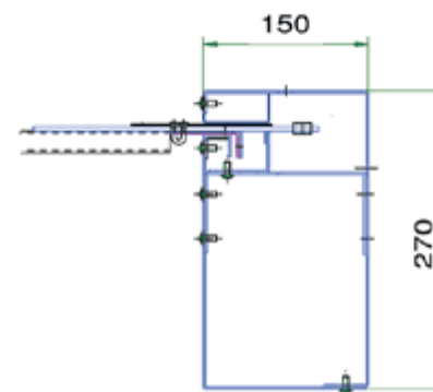
Направляющая шина
